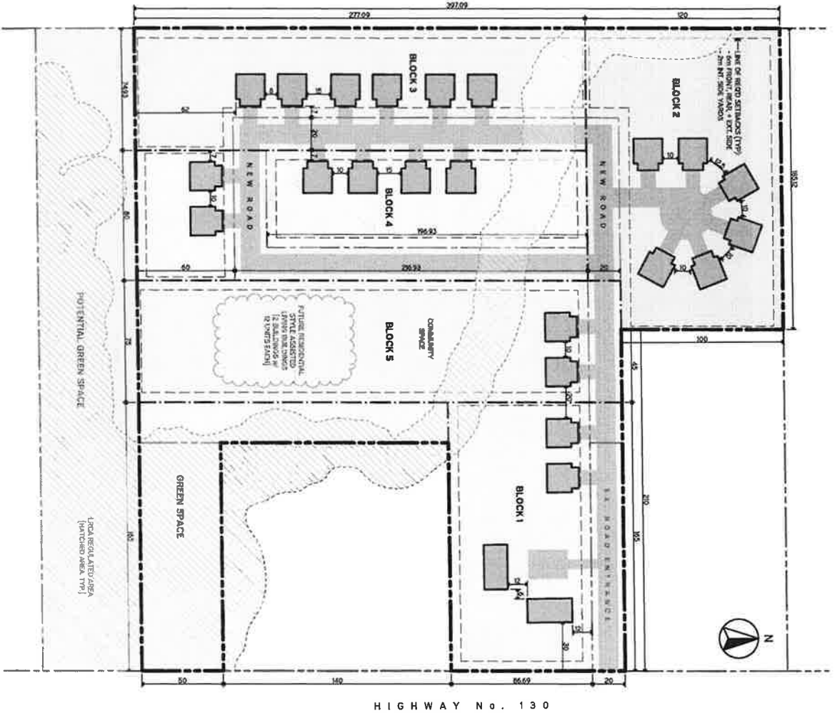
SITE PLAN SCALE: 1:2000
